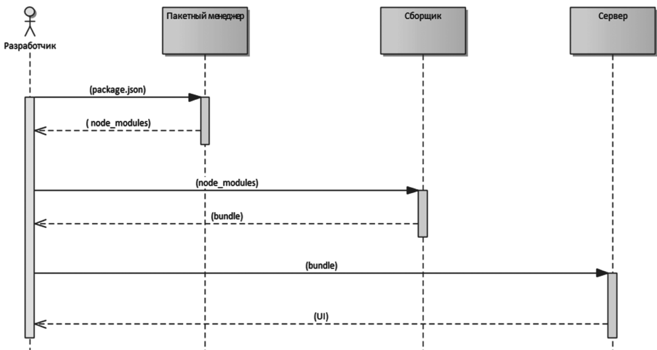
Рис. 1. Диаграмма последовательностей процесса
