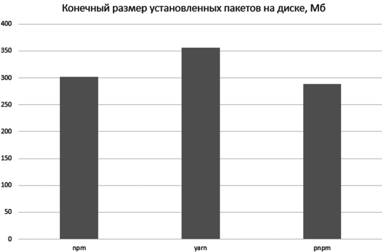
Рис. 8. Сравнение конечного размера дерева зависимостей
