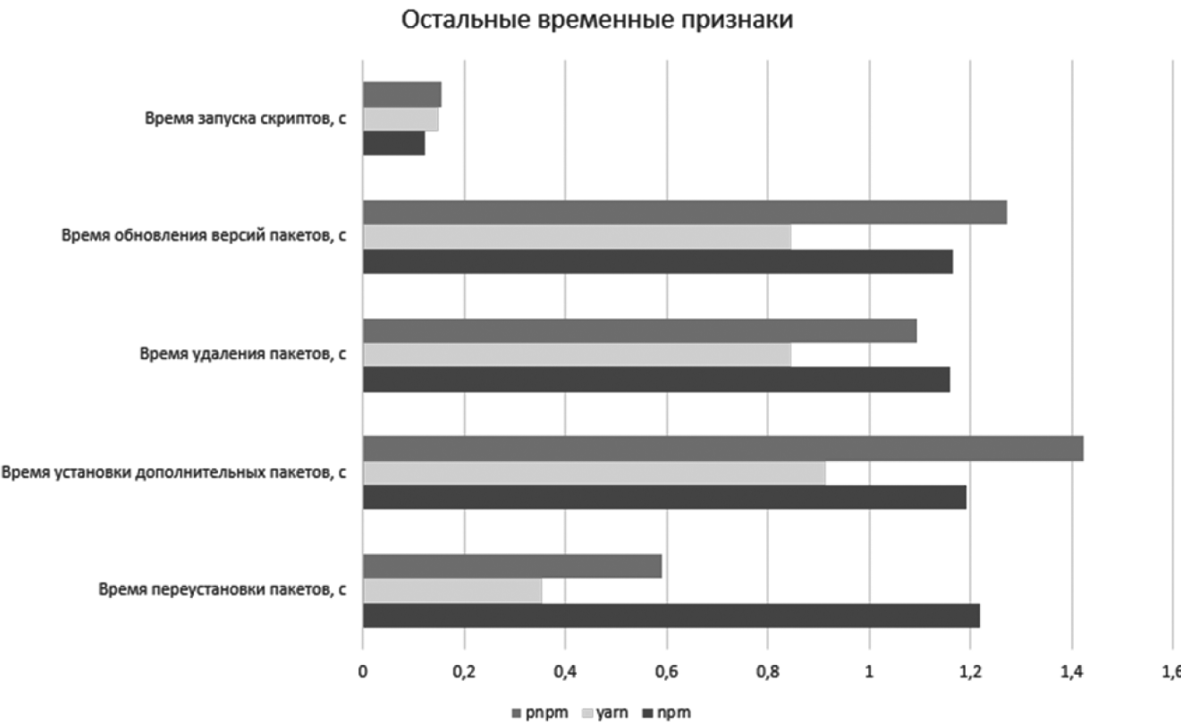
Рис. 9. Сравнение остальных временных признаков
