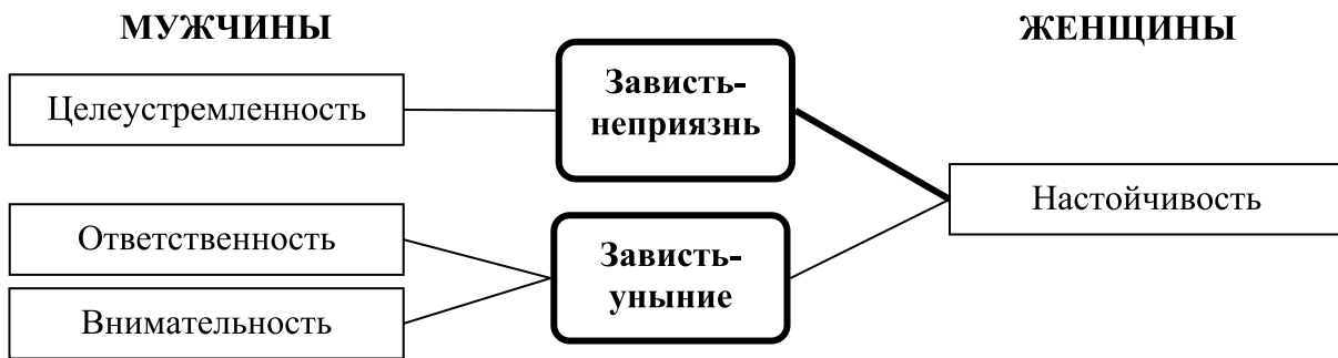
Рис. 2. Корреляции видов зависти с волевыми характеристиками у мужчин и женщин. Примечание: Сплошная линия — прямая связь, пунктирная линия — обратная связь; толщина линии показывает значимость связи.
