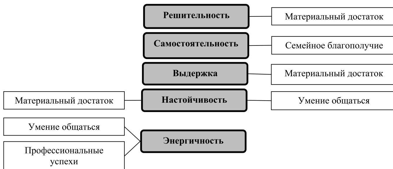
Рис. 3. Корреляции интегративного показателя зависти с волевыми характеристиками (гендерный аспект). Примечание: Пунктирная линия свидетельствует об обратной связи, а толщина линии — о значимости связи.
