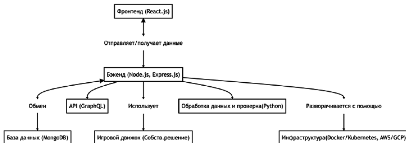
Рис. 1. Архитектура платформы
